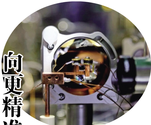
10 月 5 日在清华大学实验室拍摄的核光钟实验装置核心区域。 新华社发
